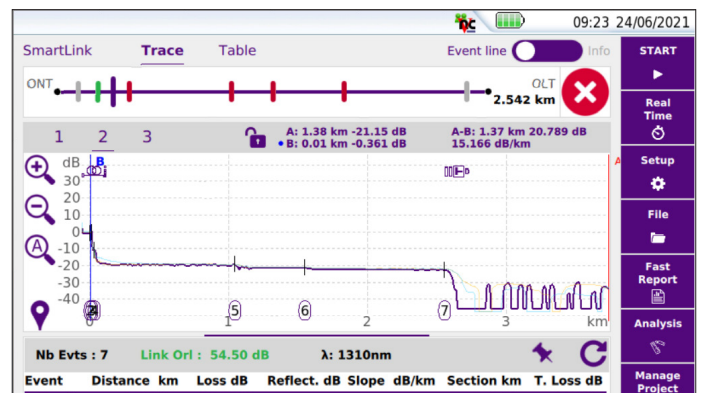
OTDR 跟踪视图
