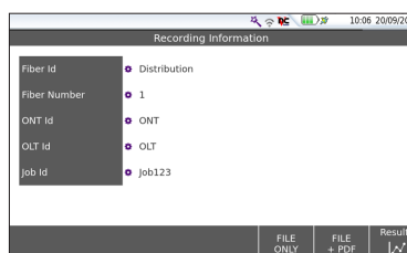
4 使用 PON 标准命名约定 (.sor 和/或 .pdf 格式) 记录测试结果
