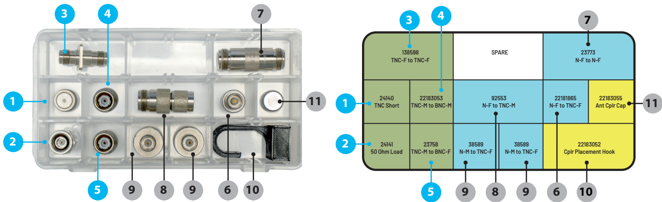
Рисунок 1. Комплект адаптера
