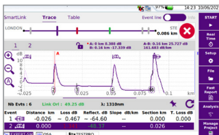
OTDR 트레이스 뷰
