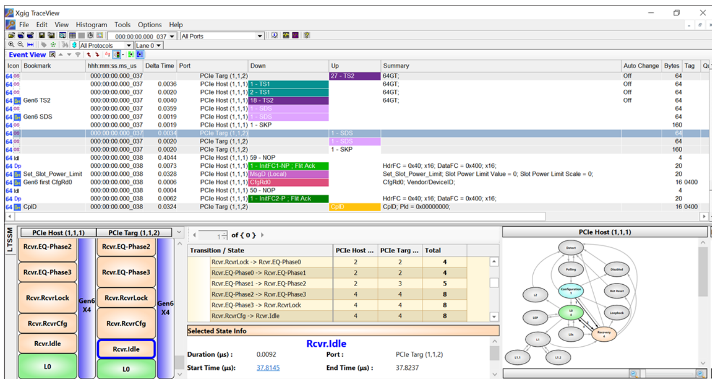
図 2 - Xgig アナライザを使った PCIe6 トレースキャプチャ
